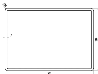
TABLICA REJESTRACYJNA SAMOCHODOWA DWURZĘDOWA
