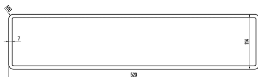
TABLICA REJESTRACYJNA SAMOCHODOWA JEDNORZĘDOWA
